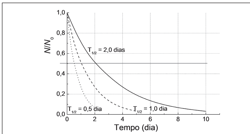
Figura 2 – Curva teórica de decaimento relativo para amostras com meia-vida de 0,5 dia, 1,0 dia e 2,0 dias. A intersecção entre cada curva e a reta cinza traçada horizontalmente no valor de N/N_0 = 0,5 fornece no eixo das abcissas a meia-vida de cada amostra.
